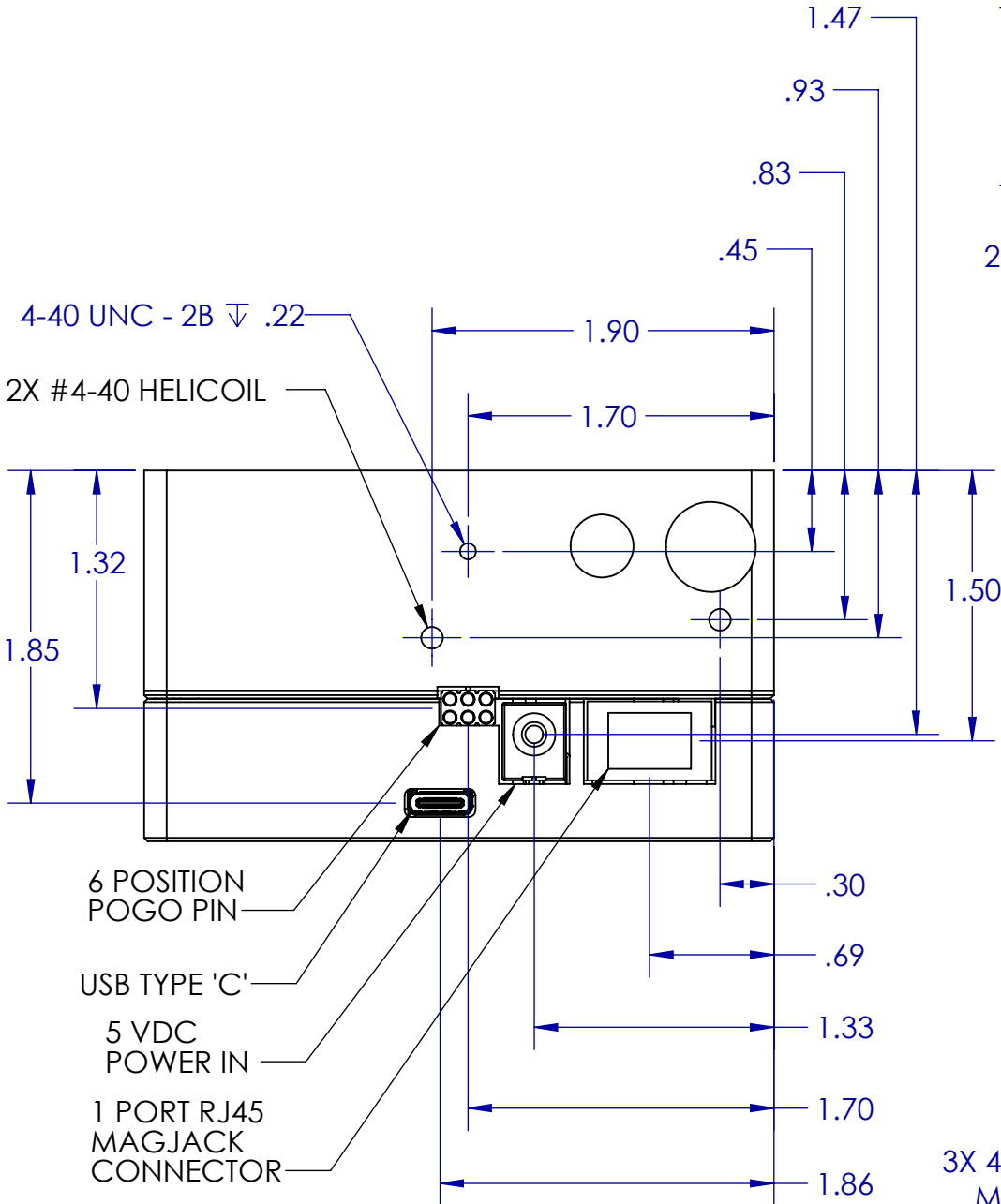
VIEW A-A
